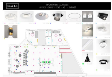
EXEMPLE D'IMPLANTATION D'ÉCLAIRAGES
